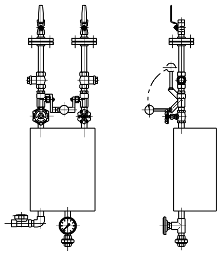
熱交換式タンデム型給湯器
