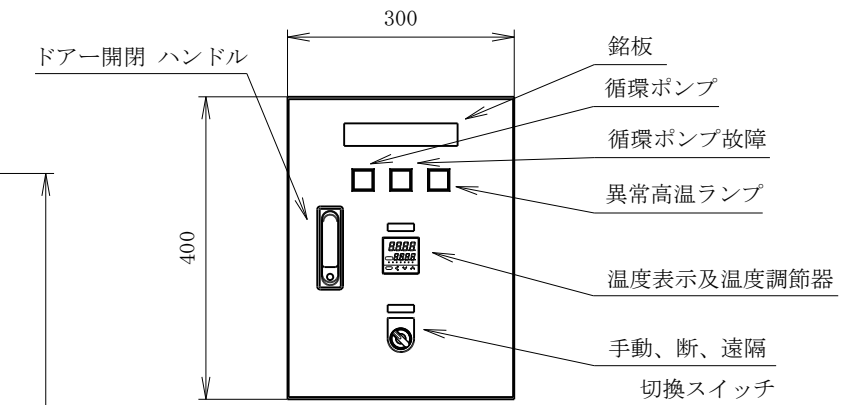
制御盤
