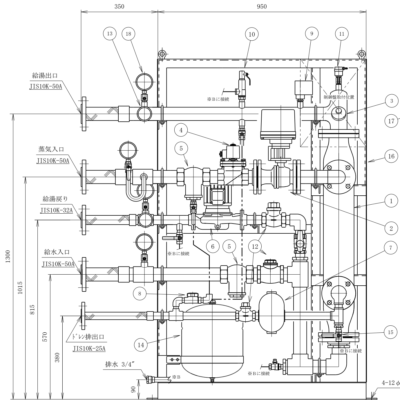
A-A' 矢視
