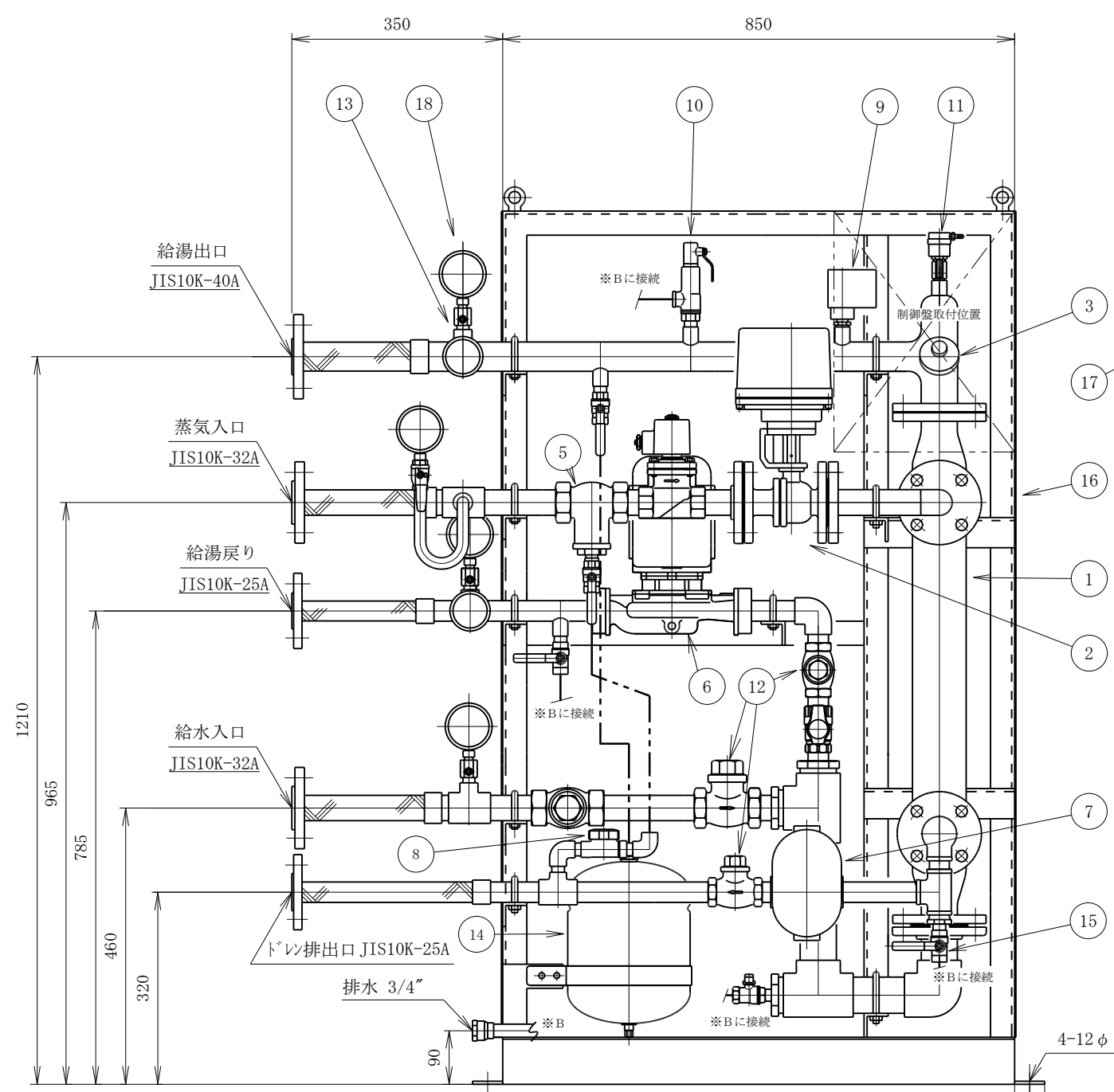
A-A' 矢視
