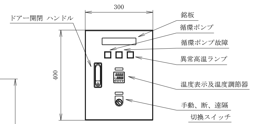
制御盤
