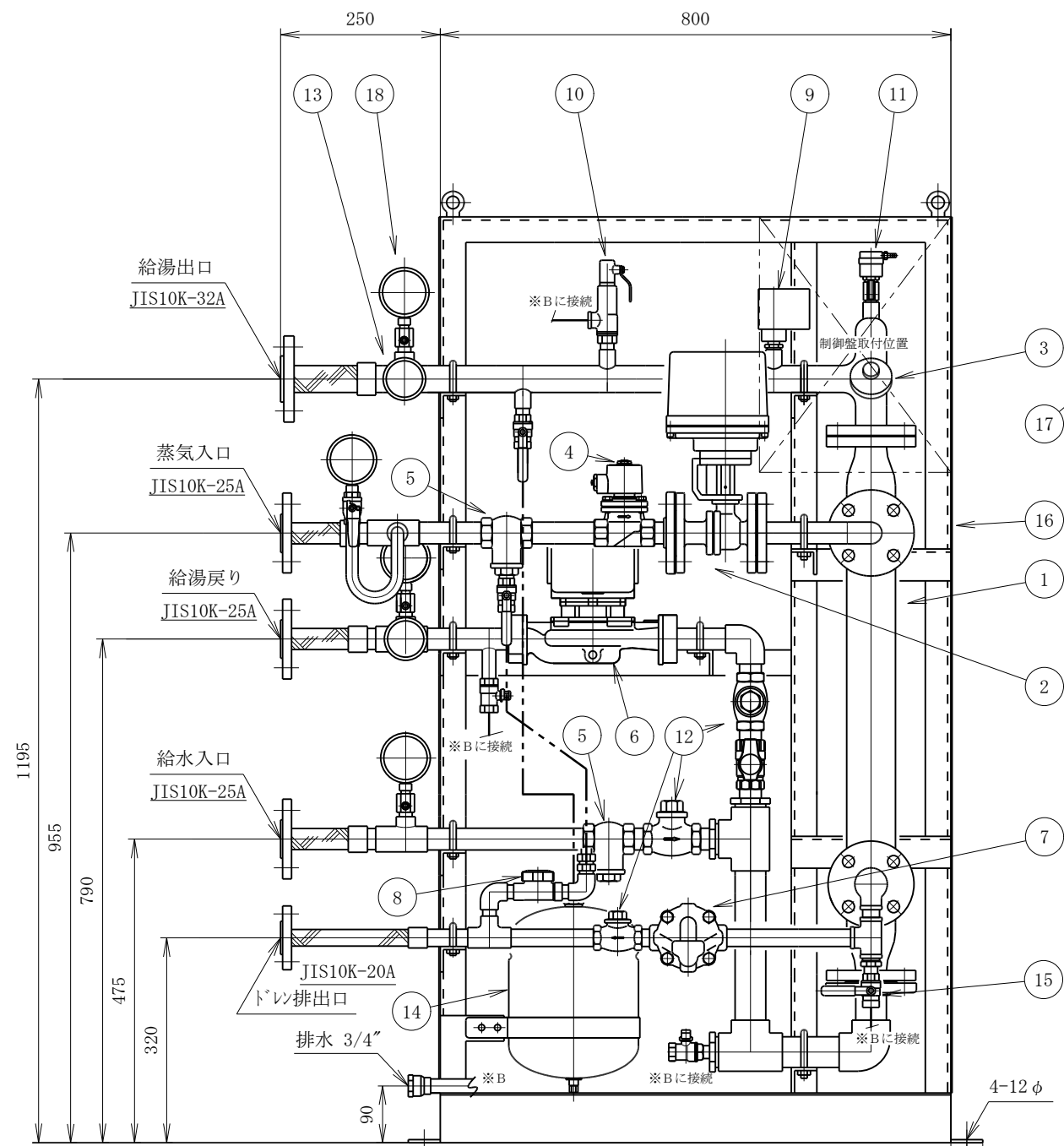
A-A' 矢視
