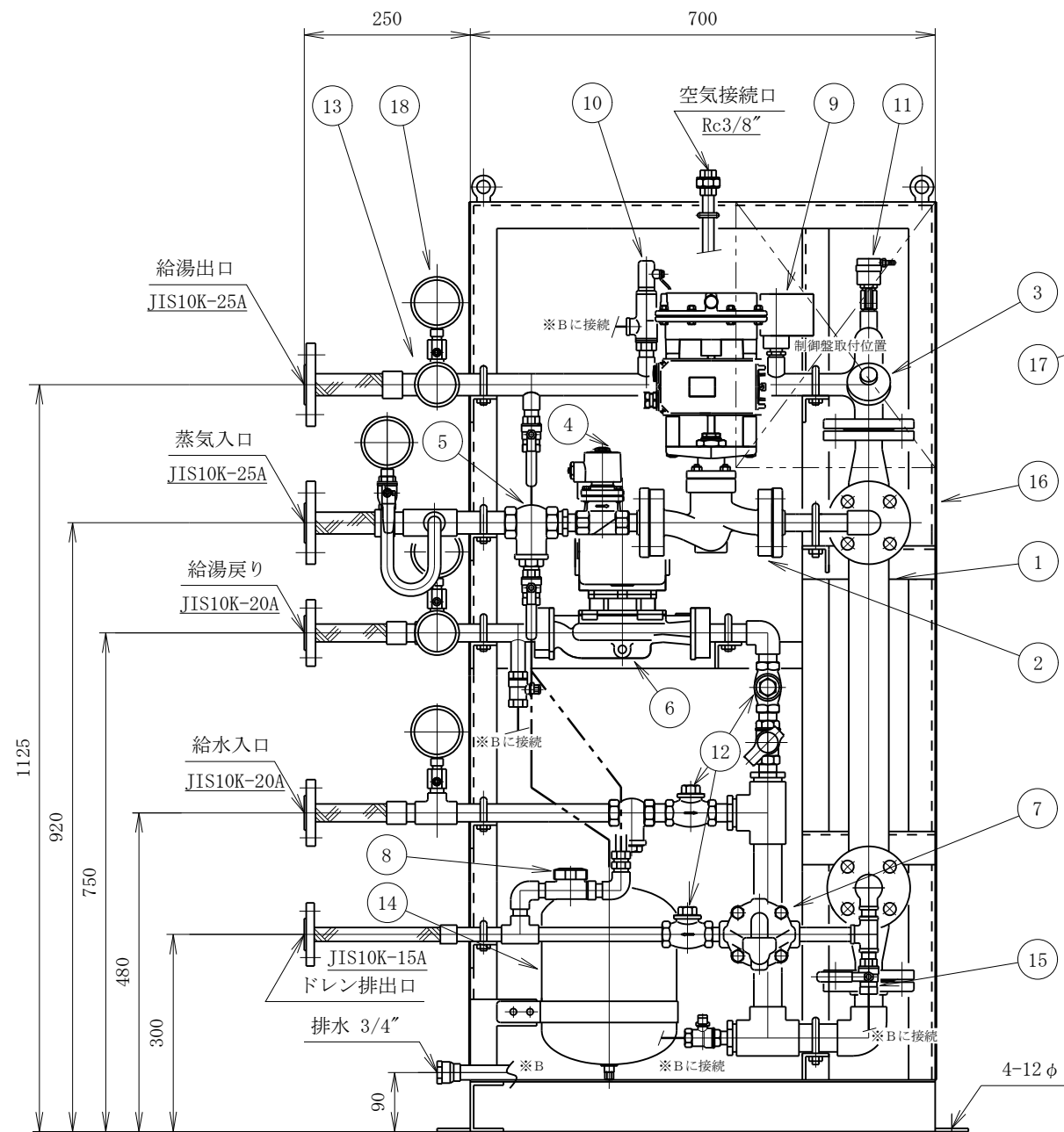
A-A' 矢視
