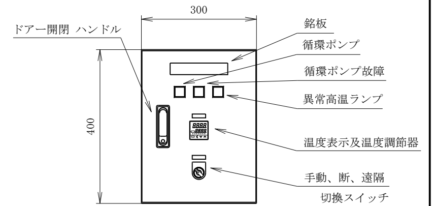
制御盤
