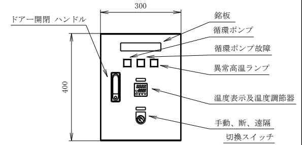
制御盤
