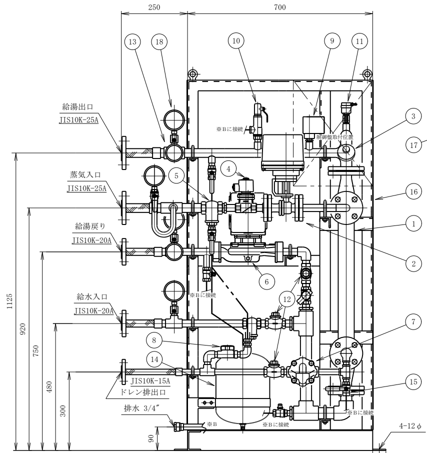
A-A' 矢視
