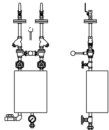
熱交換式タンデム型給湯器
