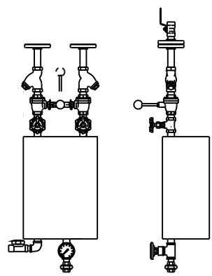
熱交換式タンデム型給湯器
